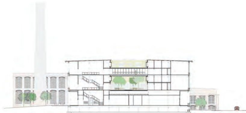
A SECTION SCALE: 1/16" = 1'-0"
